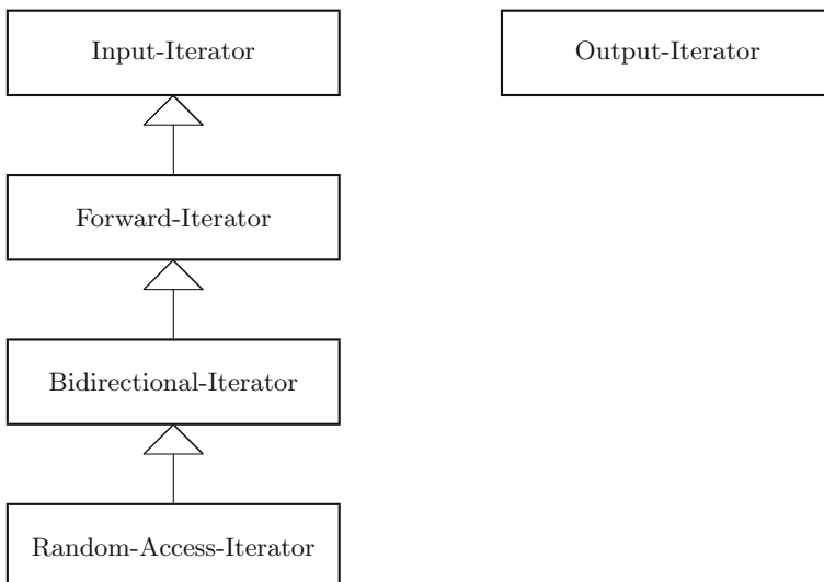
Abb. 5.4 Schematische Darstellung der Beziehungen zwischen den Iteratortypen
